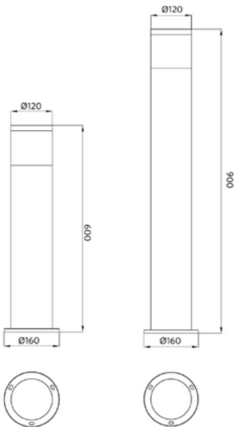
LEDBollard-P L600
