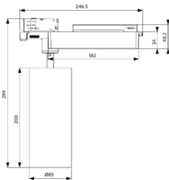
LEDspot3C-C-P 37W-BLE
