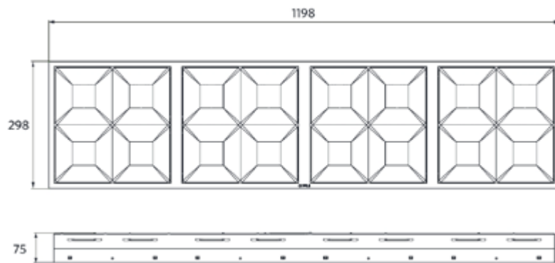
LEDPanelRc-G Re298
