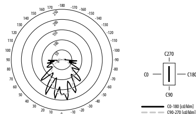
Fényeloszlási görbe
